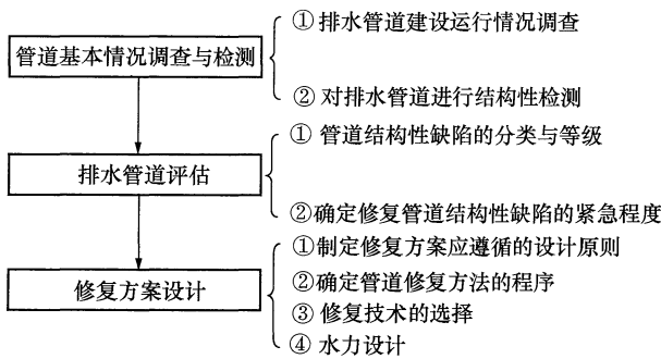
图 4 制定排水渠修复方案程序
