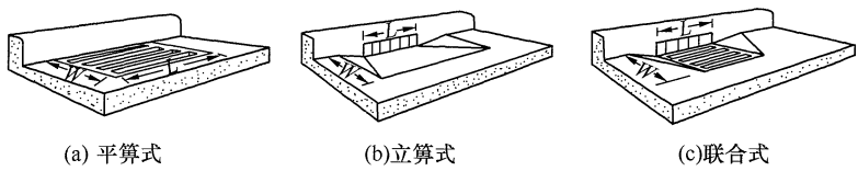
图 1 雨水算布置类型图
