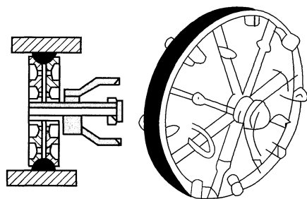
图 3 机械管塞
