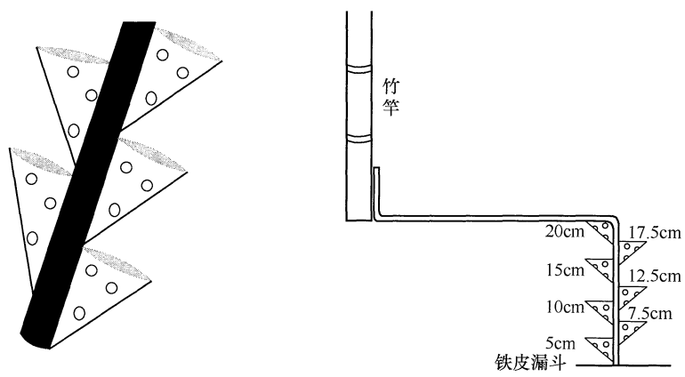
图 2 量泥斗测量泥深示意
